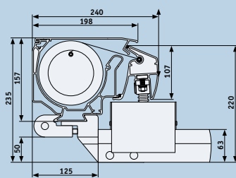
Kastenschnitt
