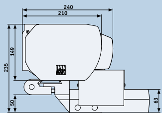
Seitenansicht
